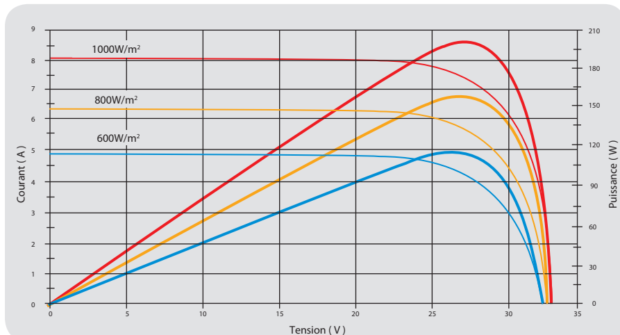
Courbe courant-tension et puissance-tension (200W)
